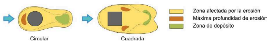
FIGURA 4.5.- COMPONENTES DE LA EROSIÓN CUANDO LAS DIMENSIONES DE LOS OBS-TÁCULOS AL PASO DE LA CORRIENTE SON PEQUEÑAS EN RELACIÓN CON EL CAUCE
