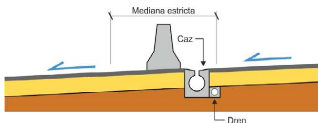
FIGURA 3.14 CAZ TIPO SUMIDERO CONTINUO EN MEDIANA ERICTA
