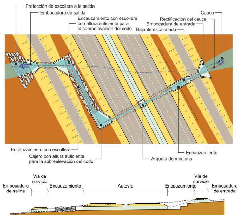
FIGURA 4.7.- EJEMPLO DE ODT COMPUESTA DE VARIOS TRAMOS.
