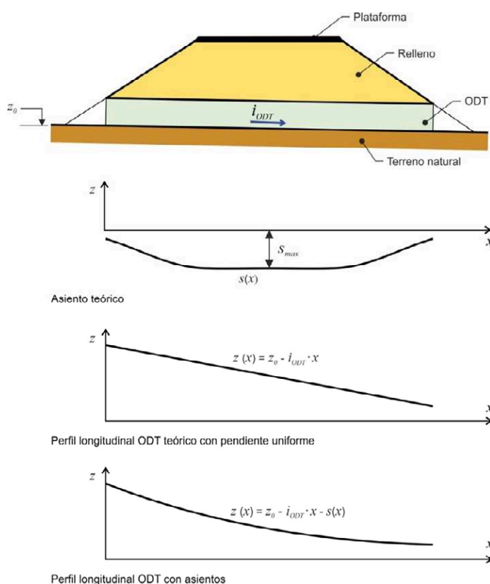
FIGURA 4.9.- CONSIDERACIÓN DE LOS ASIENTOS DEL CIMIENTO DEL RELLENO
