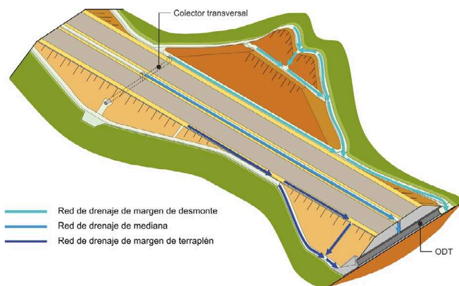
FIGURA 3.1.- EJEMPLO DE REDES DE DRENAJE DE PLATAFORMA Y MÁRGENES
