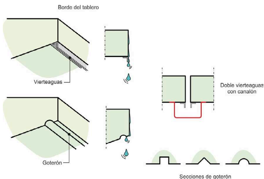
FIGURA 3.30 EJEMPLOS DE VIERTEAGUAS Y GOTERONES
