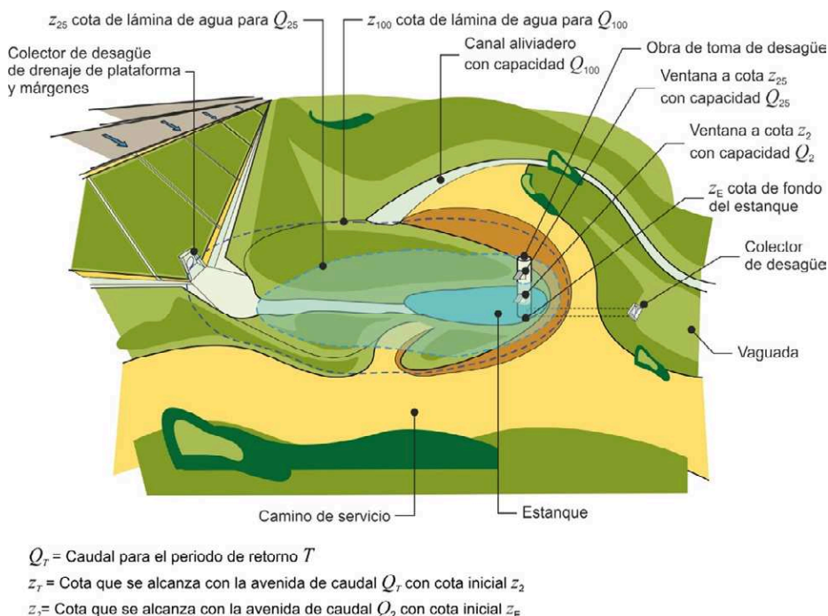
FIGURA 3.43 EJEMPLO DE ELEMENTO DE LAMINACIÓN
