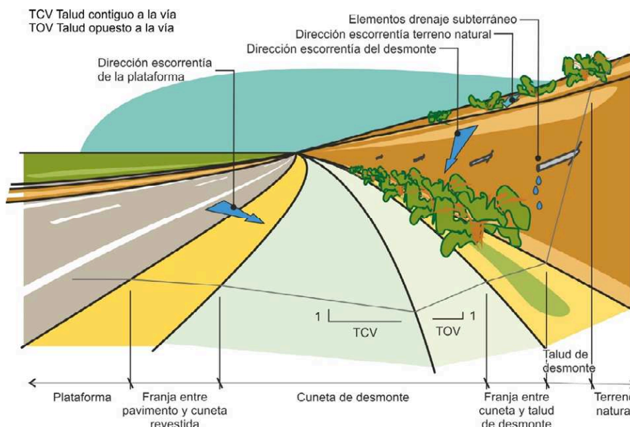
FIGURA 3.16 EJEMPLO DE CUNETA EN MARGEN DE DESMONTES
