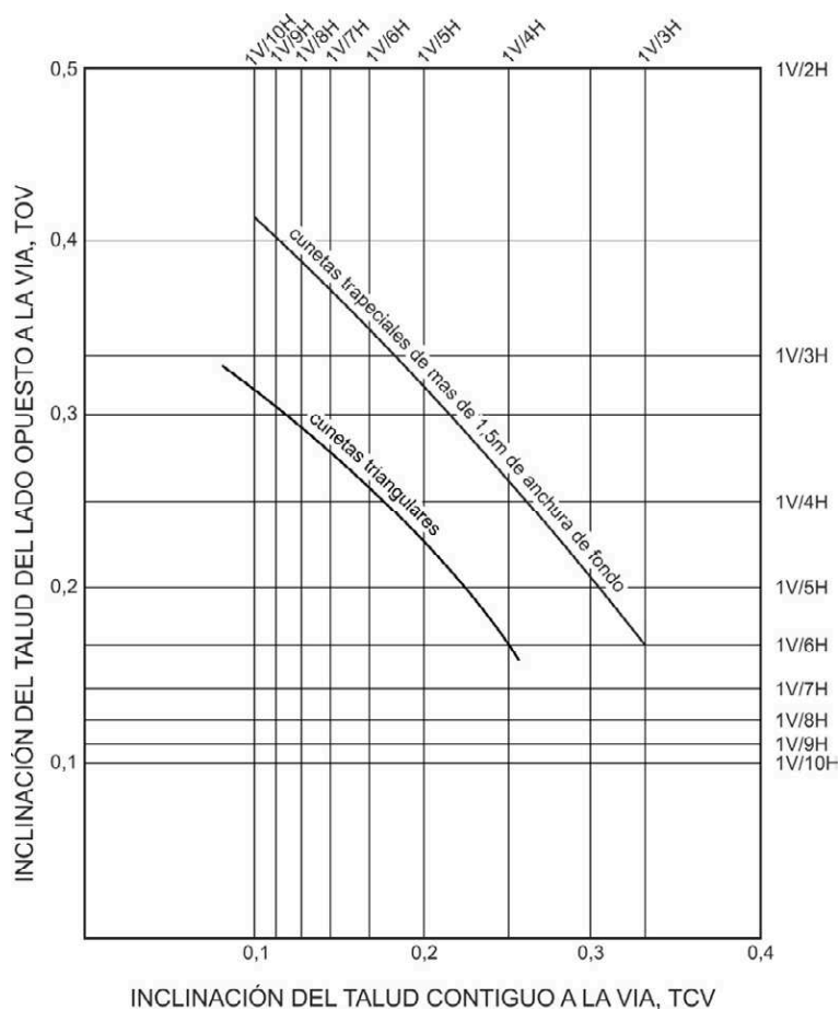
FIGURA 3.17 TALUDES DE CUNETAS EN MARGEN DE DESMONTES
