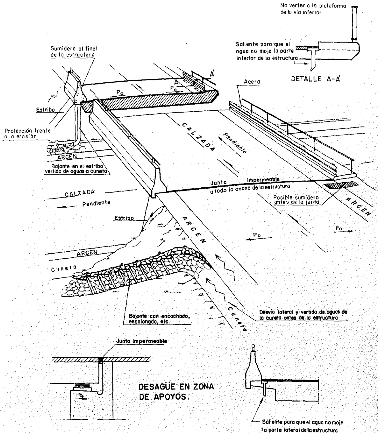
Fig. 3.8. DRENAJE EN OBRAS DE PASO
