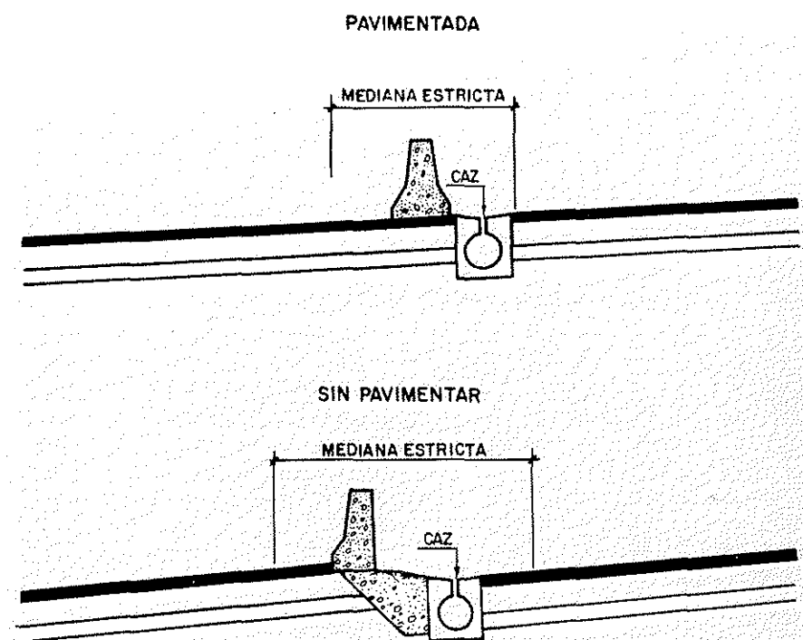
Fig. 3.3. MEDIANA Estricta EN TRAMOS CON PERALTE
