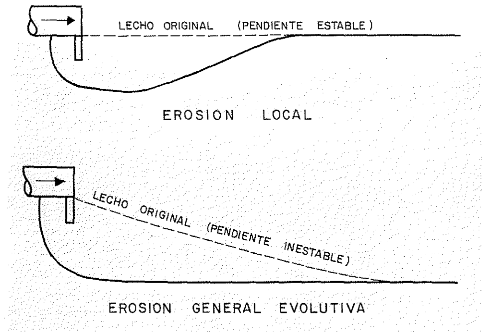
Fig. 5.16. TIPOS DE EROSION
