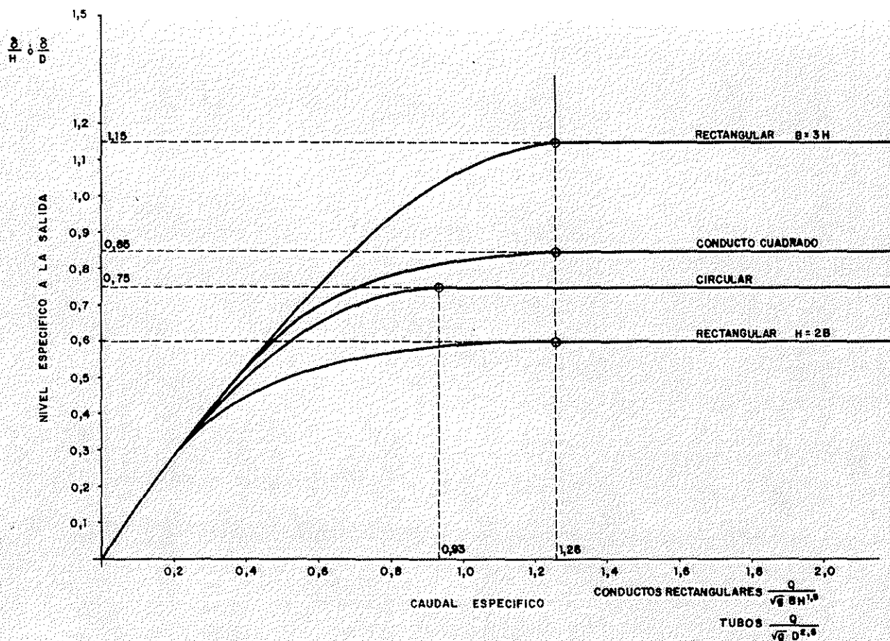
Fig. 5.19. LIMITE DE NIVELES ALTOS A LA SALIDA
