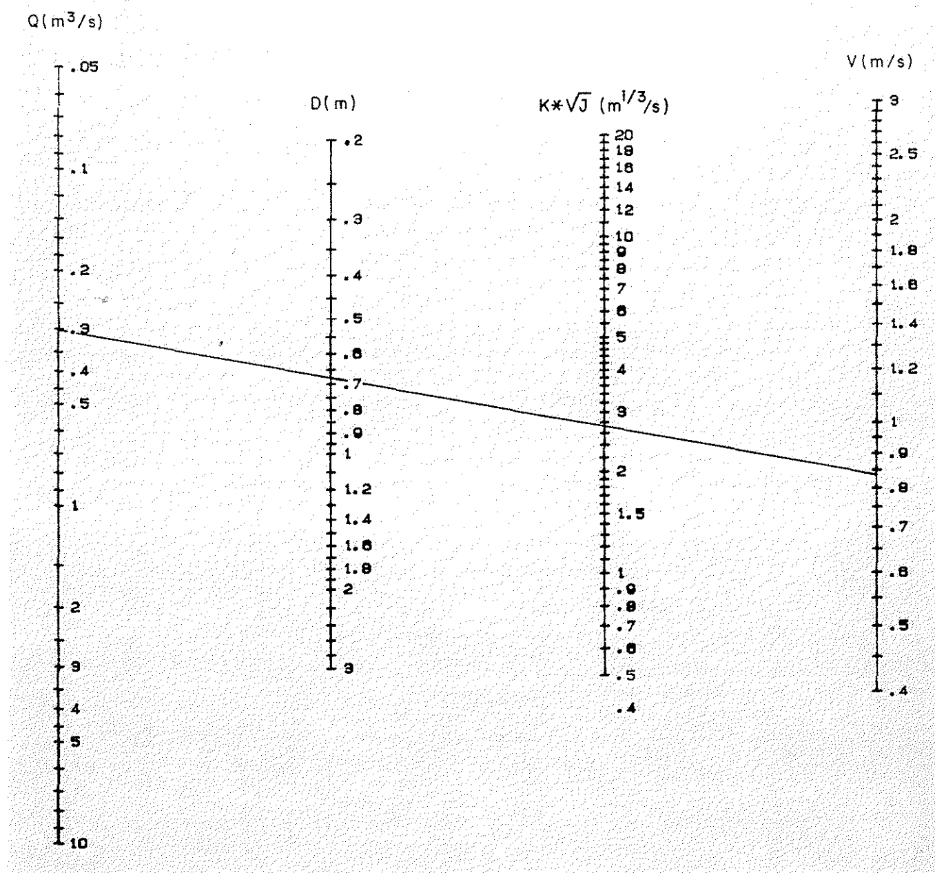
Fig. 4.3. DESAGÜE DE TUBOS EN CARGA
