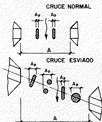
Fig. 5.5. INFLUENCIA DE LA ANCHURA Y TIPO DE PILA EN K_p
