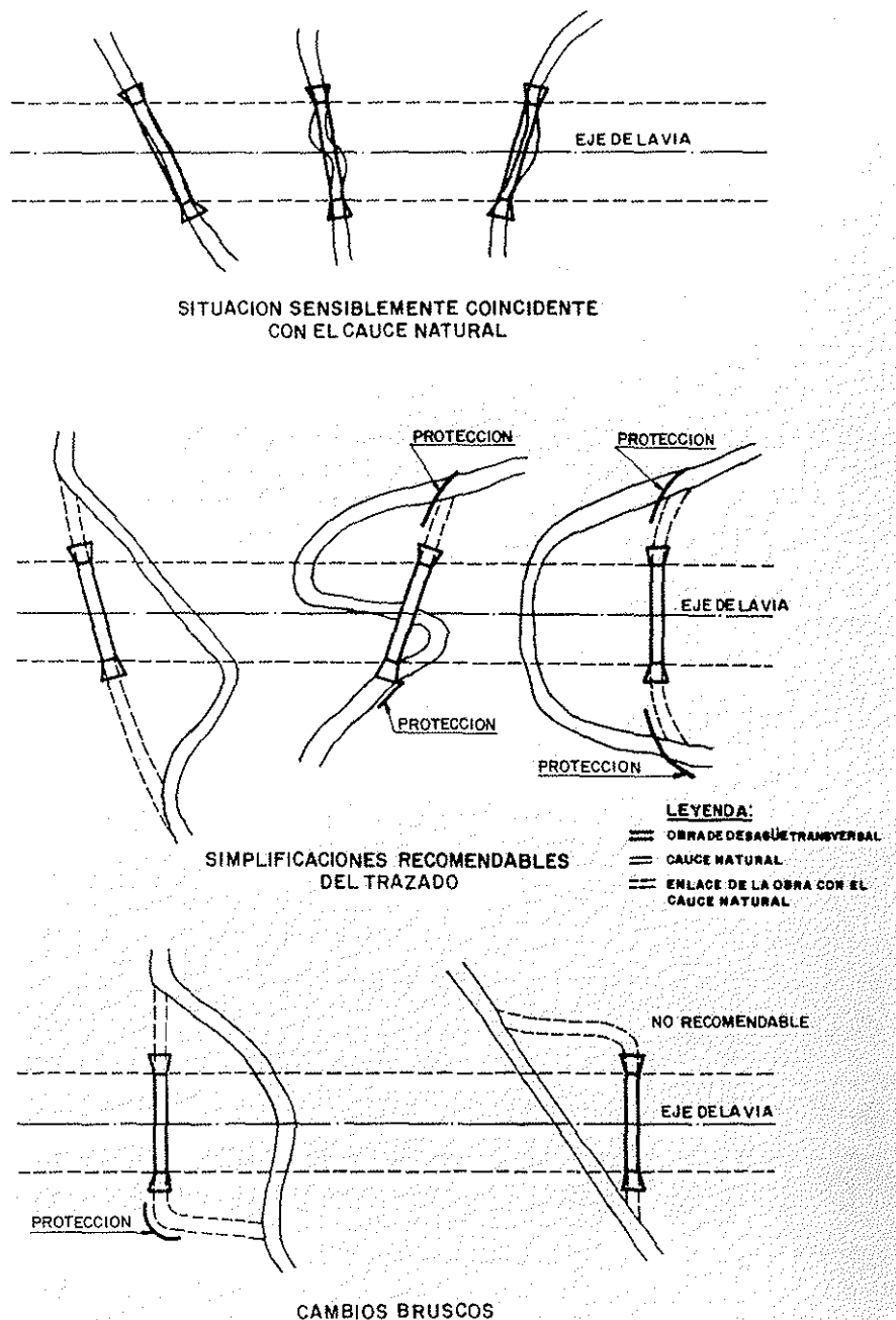
Fig. 5.1. PLANTA DE PEQUEÑAS OBRAS DE DRENAJE TRANSVERSAL
