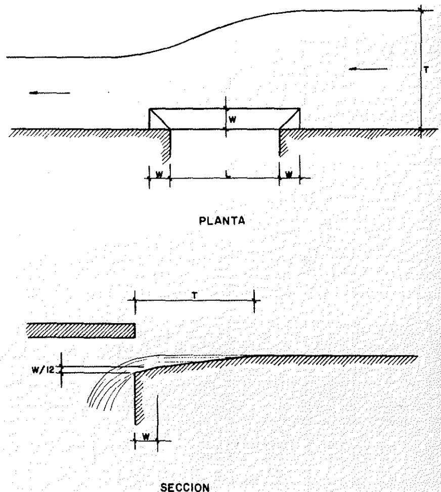
Fig. 3.13. SUMIDERO LATERAL
