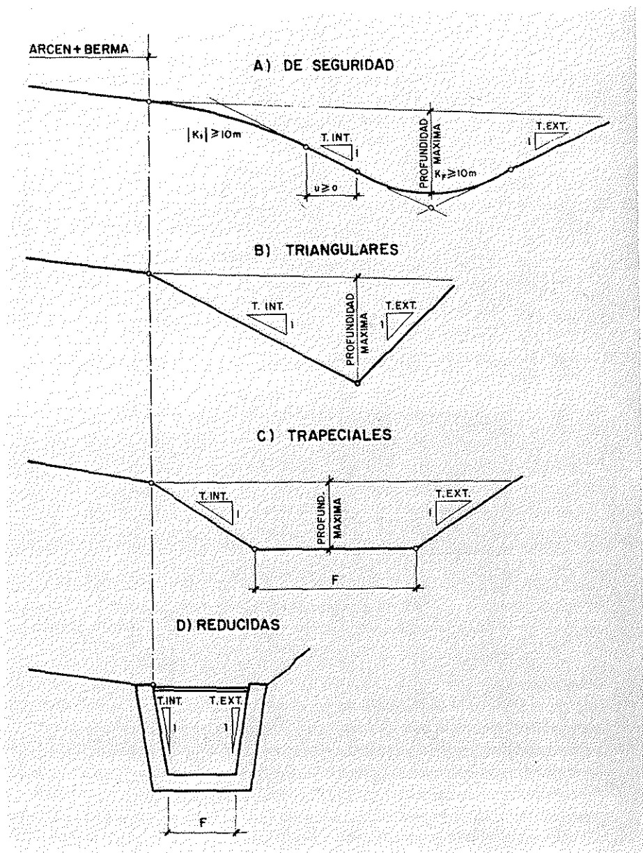
Fig. 3.10. CUNETAS
